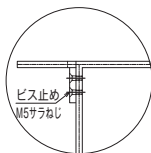
コーナー納まりの連結部詳細
