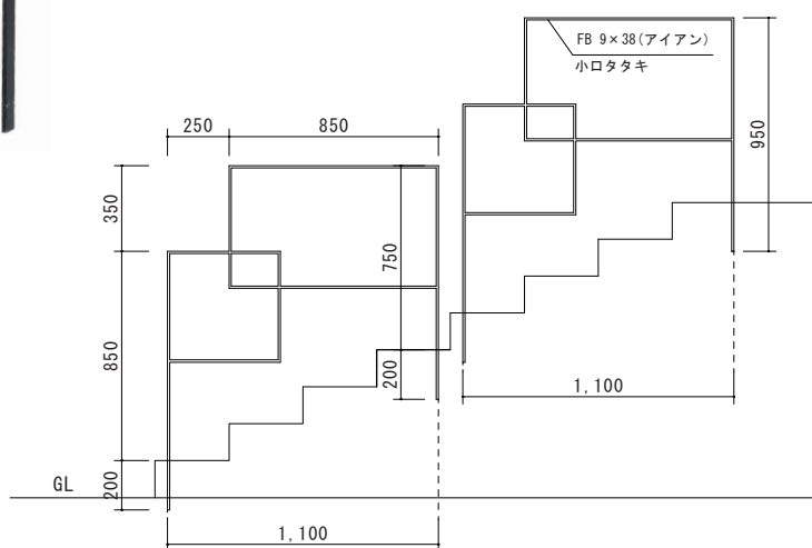
階段手摺
