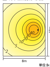
■ 床面照度分布図
