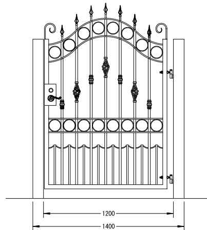
門扉-D型 M8995 (片開き+柱仕様) ¥810,000(参考価格) W1200mm×H1800mm
