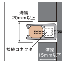
壁面上に設置する場合、溝を設けて固定具Bを取り付けることにより結線スペースを隠し、きれいに取ることが出来ます(溝幅や狭かつ溝が深いとラインライトが外せないでください)。
