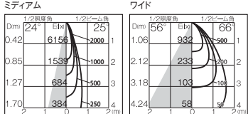
ビーム球150Wクラス
