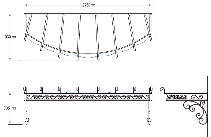
キャンピアー(庇)ーB型
