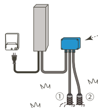
⚠ ラインライト・直流電源装置・分岐ボックスは、水浸ししないような位置や場所に設置下さい。
