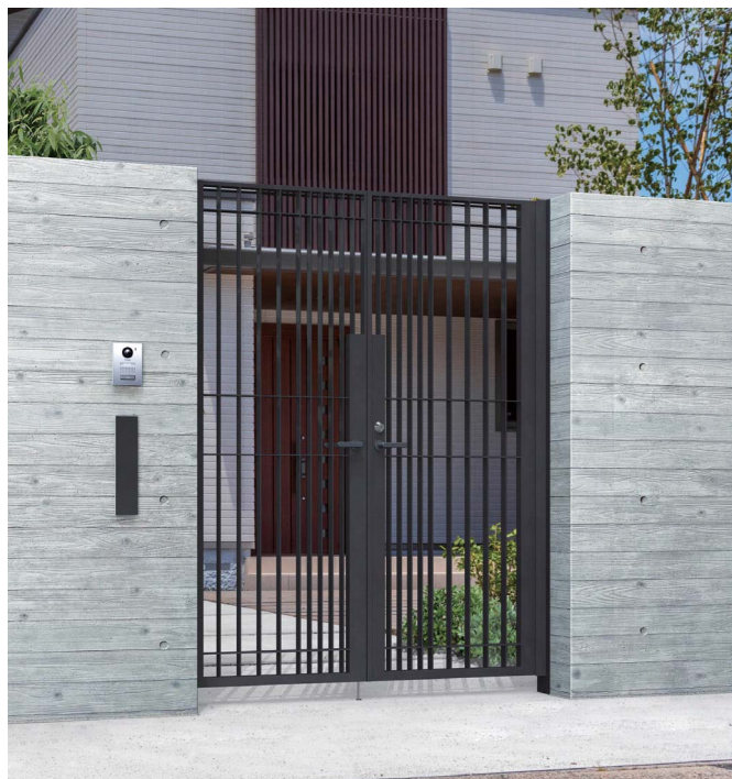
門扉② □片開き ¥659,500~/枚(参考価格) W1000×H2200~2600mm(埋め込み400mm含む) □両開き ¥1,027,000~/セット(参考価格) W1900×H2200~2600mm(埋め込み400mm含む) ※電気錠仕様の対応が可能になります。
