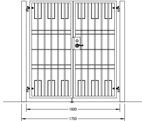
門扉-C型 M8995 (両開き+柱仕様) ¥1,000,000(参考価格) W1600mm×H1600mm
