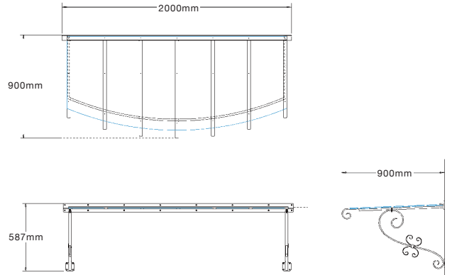
キャノピー(庇)ーC型
