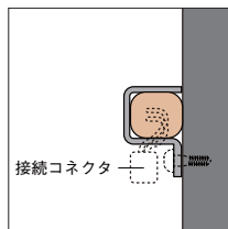
固定具 B 配線部のみ隠して灯体を露出させる 施工におすすめです。
