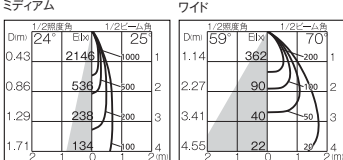
ダイクロハロゲン(JDR)75Wクラス
