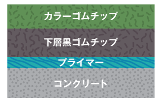
下層黒ゴムチップ厚20mmと 表層カラーゴムチップ厚10mmの 施工イメージ
