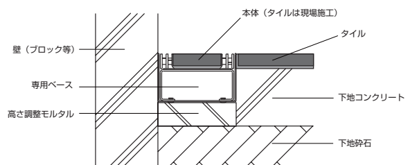
壁際に施工する場合
