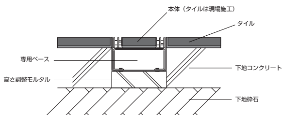
テラス中央に施工する場合
